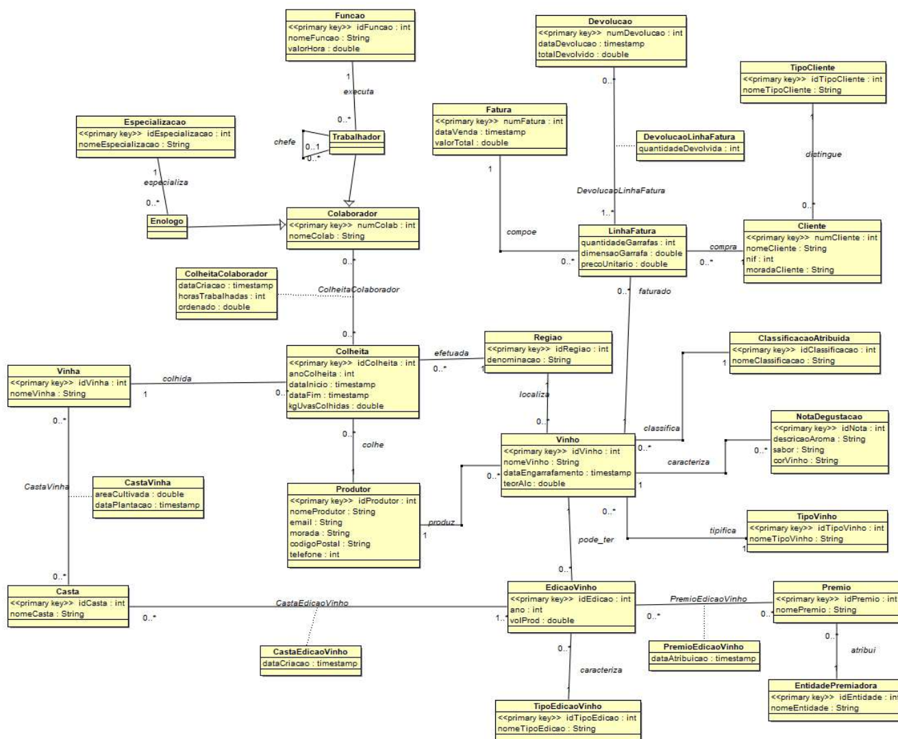
Figura 1 - Diagrama de Classes sistema “VINISYS”.
